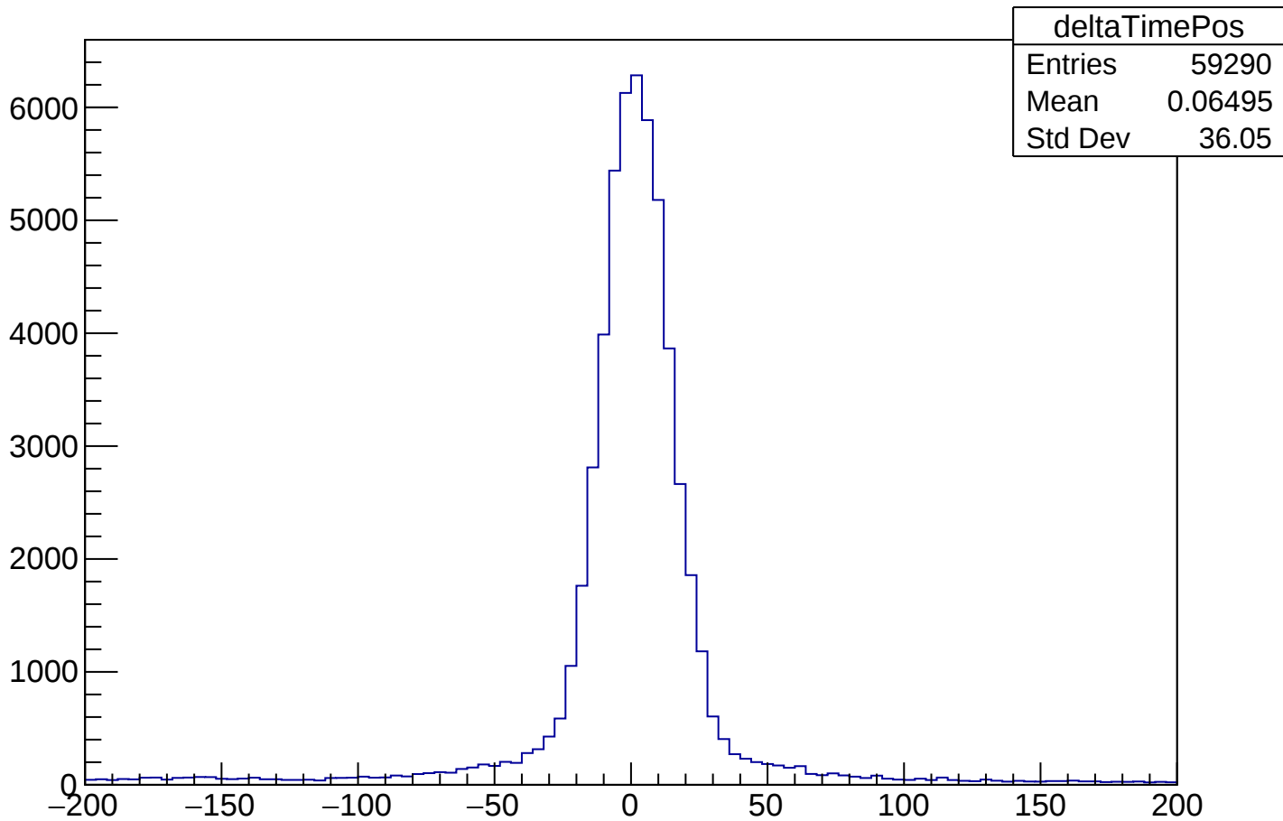
deltaTimePos
