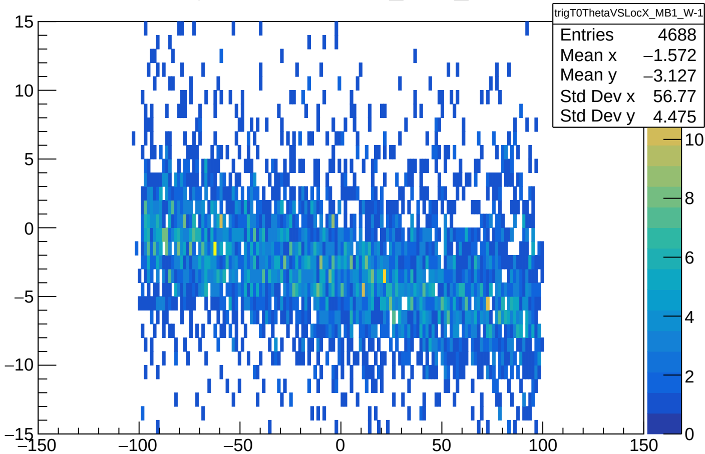
trigT0ThetaVSLocX_MB1_W-1
