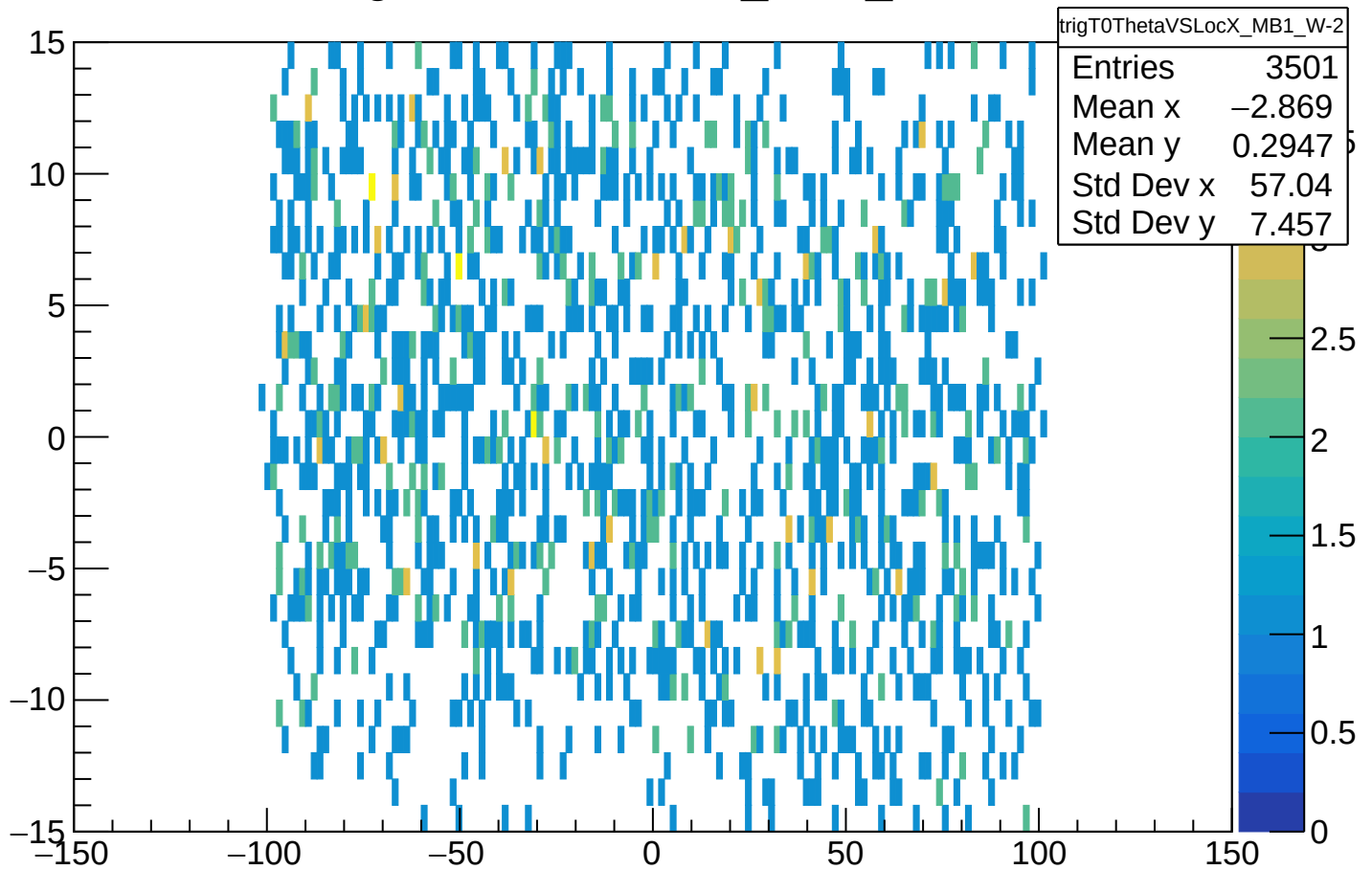
trigT0ThetaVSLocX_MB1_W-2
