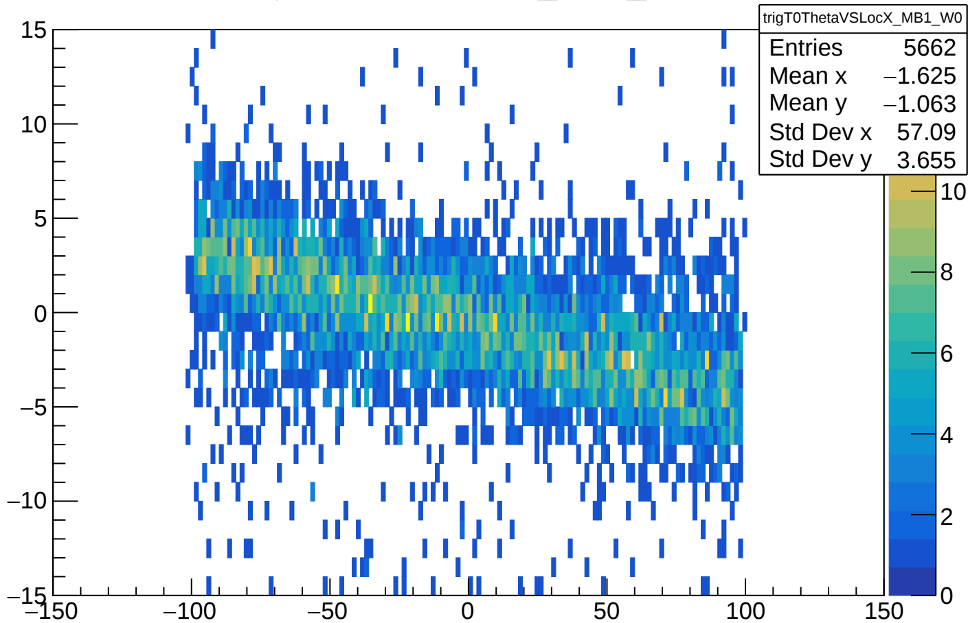
trigT0ThetaVSLocX_MB1_W0
