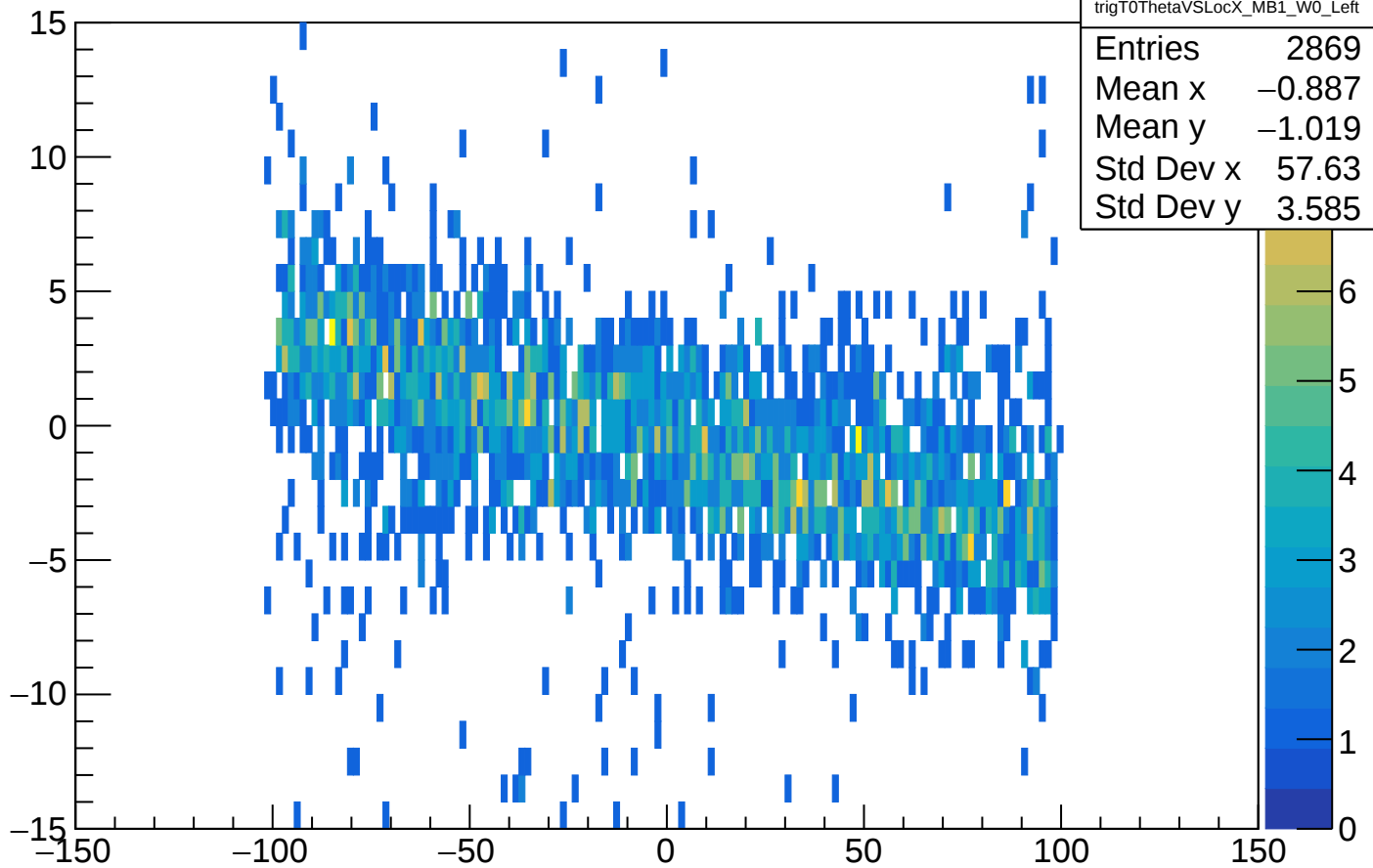
trigT0ThetaVSLocX_MB1_W0_Left
