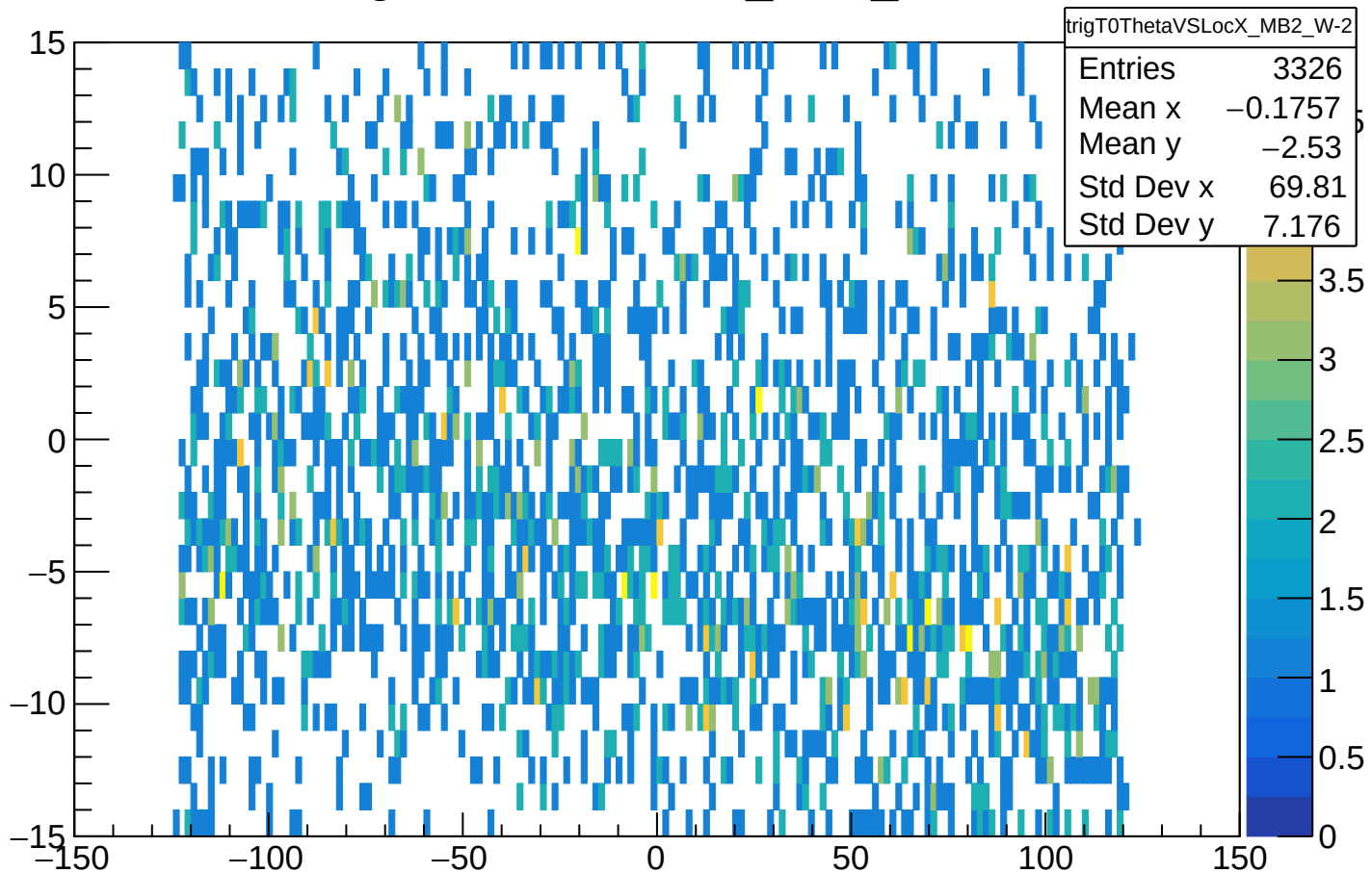
trigT0ThetaVSLocX_MB2_W-2
