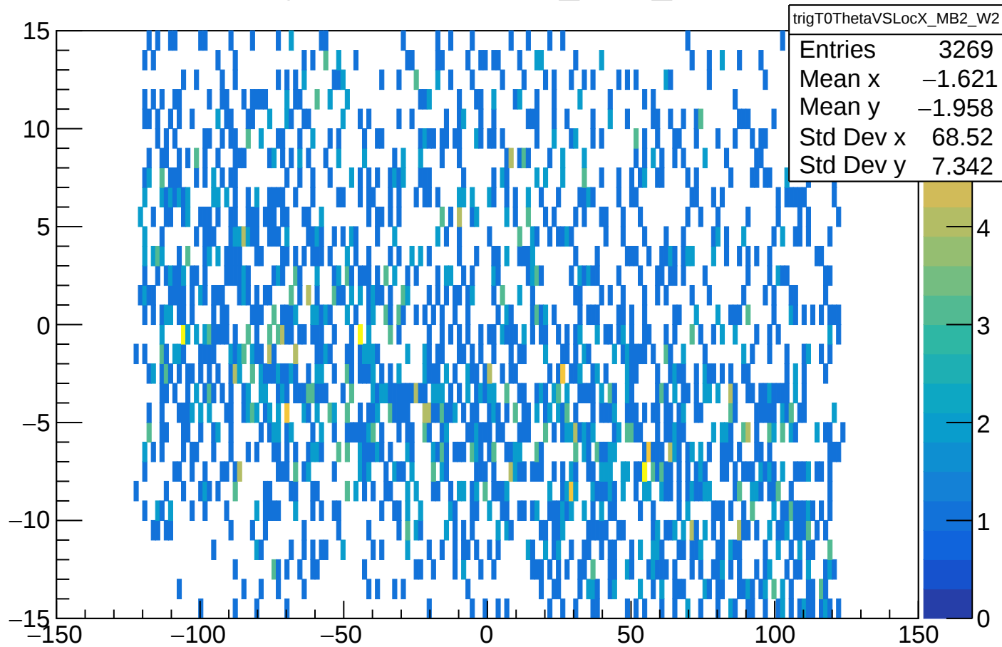
trigT0ThetaVSLocX_MB2_W2
