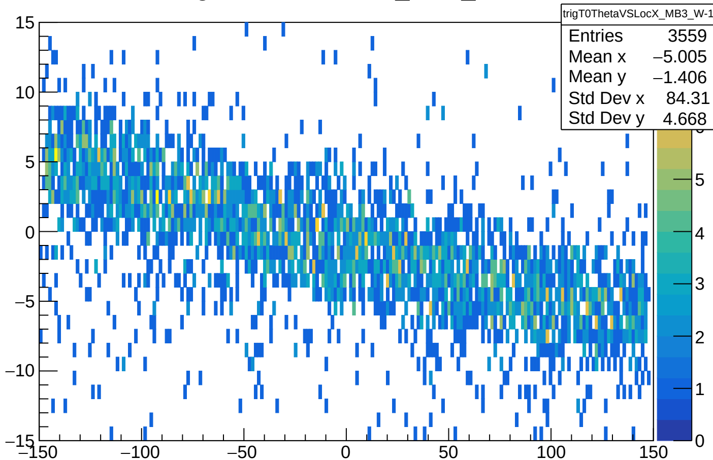
trigT0ThetaVSLocX_MB3_W-1
