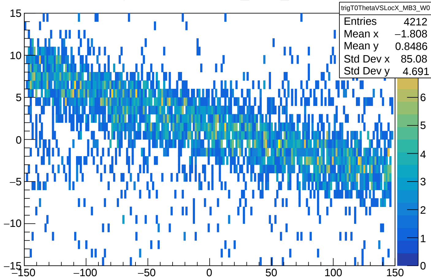
trigT0ThetaVSLocX_MB3_W0
