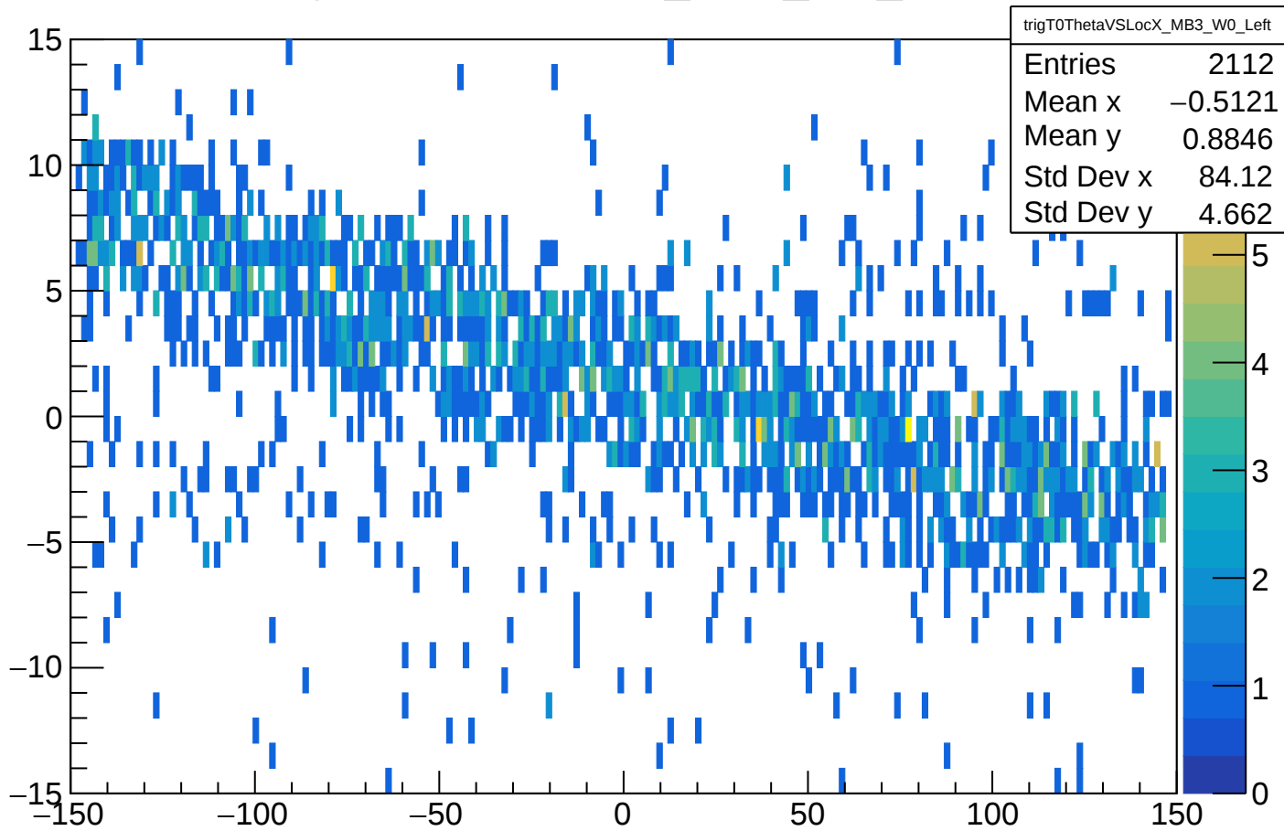
trigT0ThetaVSLocX_MB3_W0_Left
