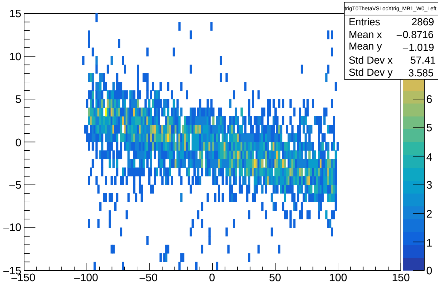
trigT0ThetaVSLocXtrig_MB1_W0_Left
