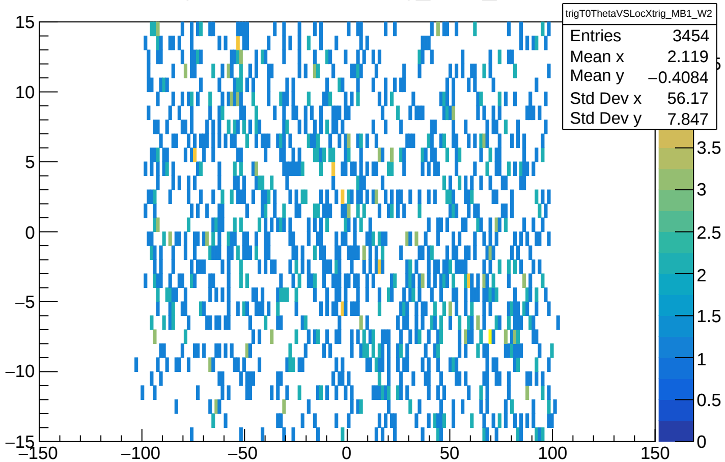
trigT0ThetaVSLocXtrig_MB1_W2
