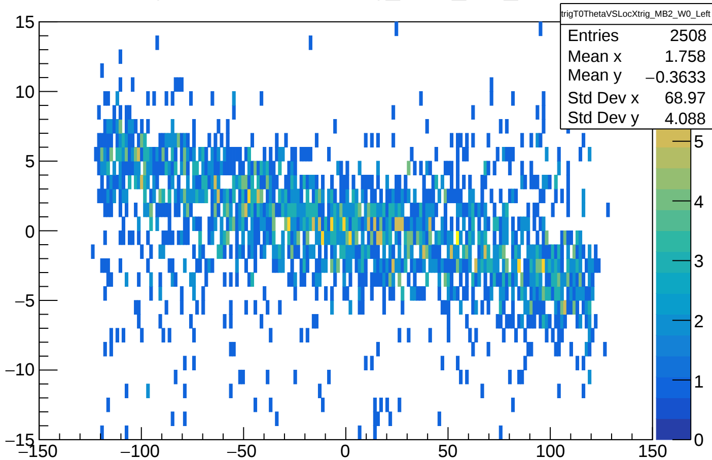
trigT0ThetaVSLocXtrig_MB2_W0_Left
