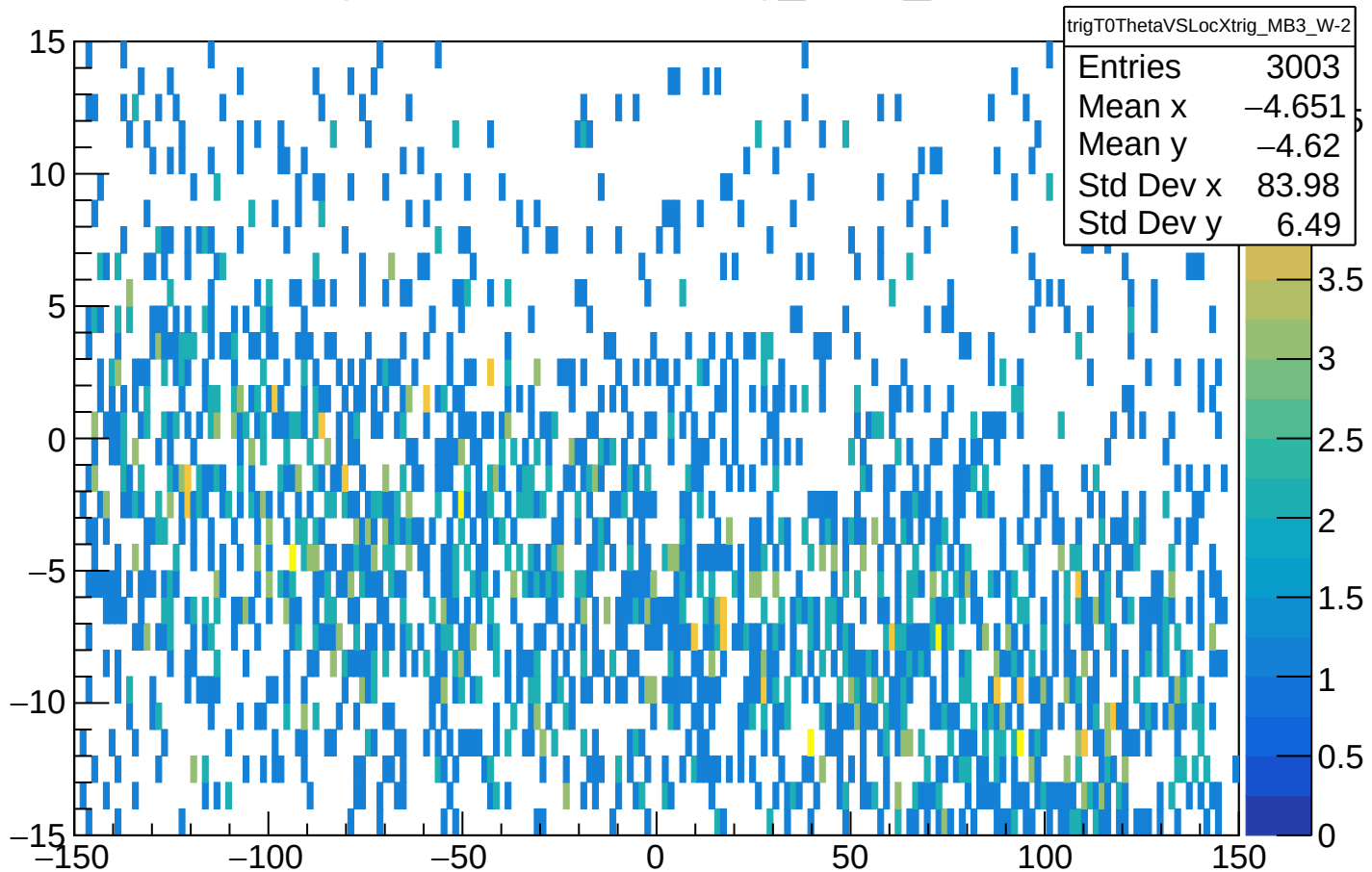
trigT0ThetaVSLocXtrig_MB3_W-2
