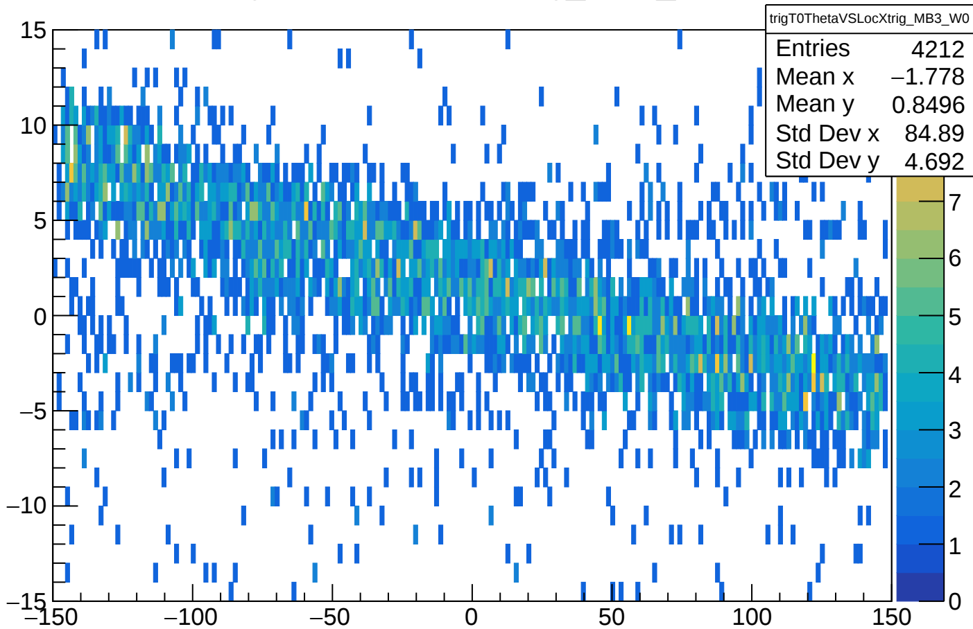
trigT0ThetaVSLocXtrig_MB3_W0
