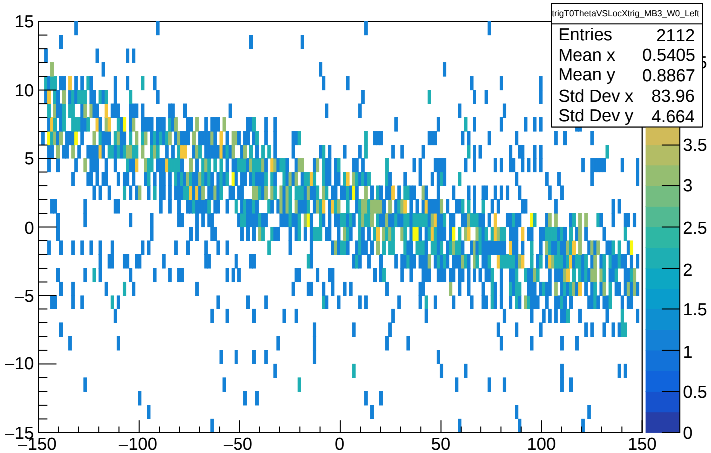
trigT0ThetaVSLocXtrig_MB3_W0_Left
