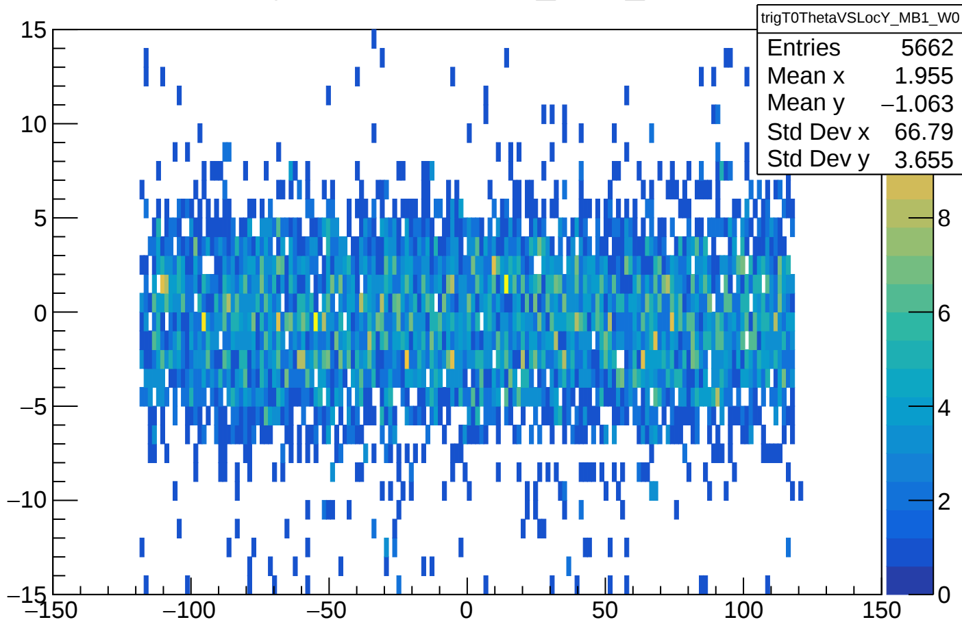
trigT0ThetaVSLocY_MB1_W0
