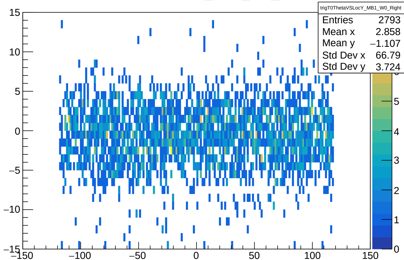
trigT0ThetaVSLocY_MB1_W0_Right
