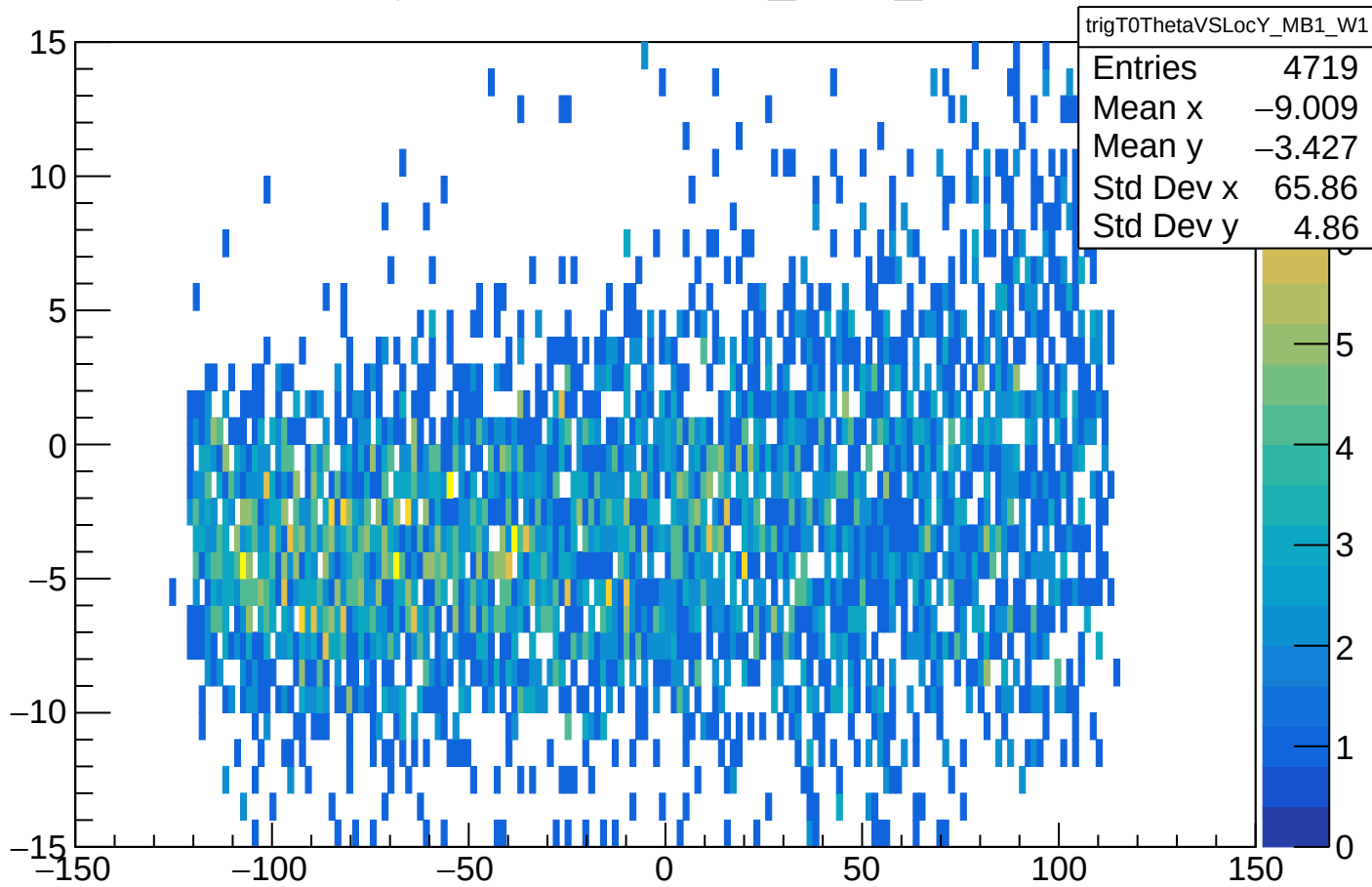
trigT0ThetaVSLocY_MB1_W1
