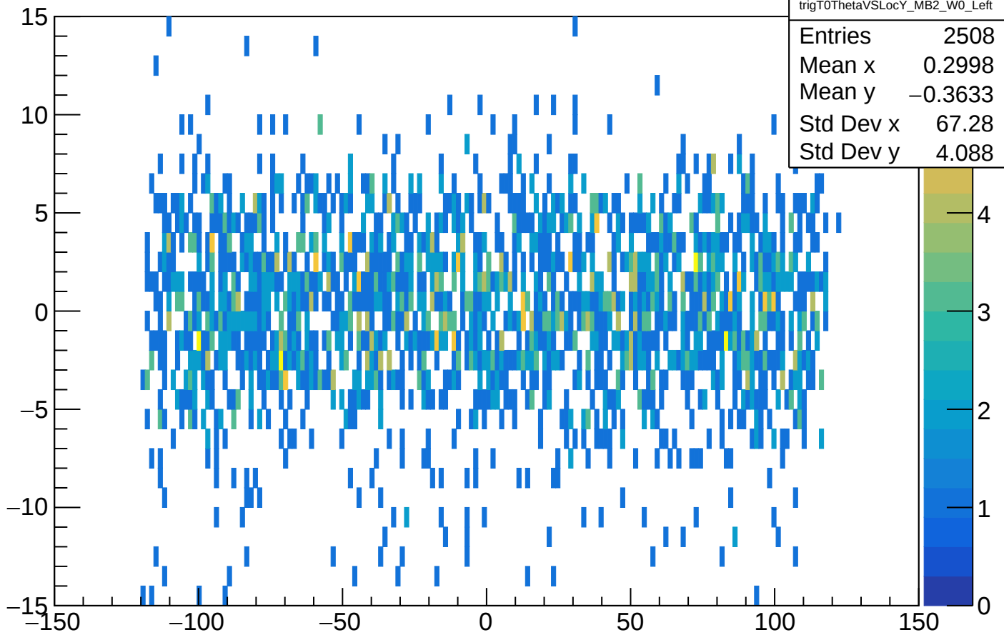
trigT0ThetaVSLocY_MB2_W0_Left
