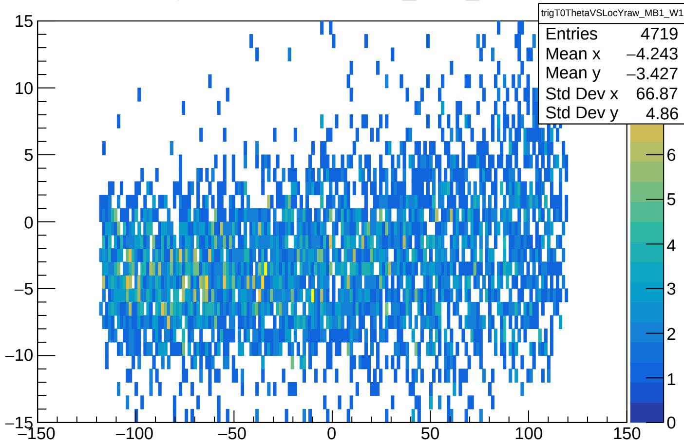
trigT0ThetaVSLocYraw_MB1_W1
