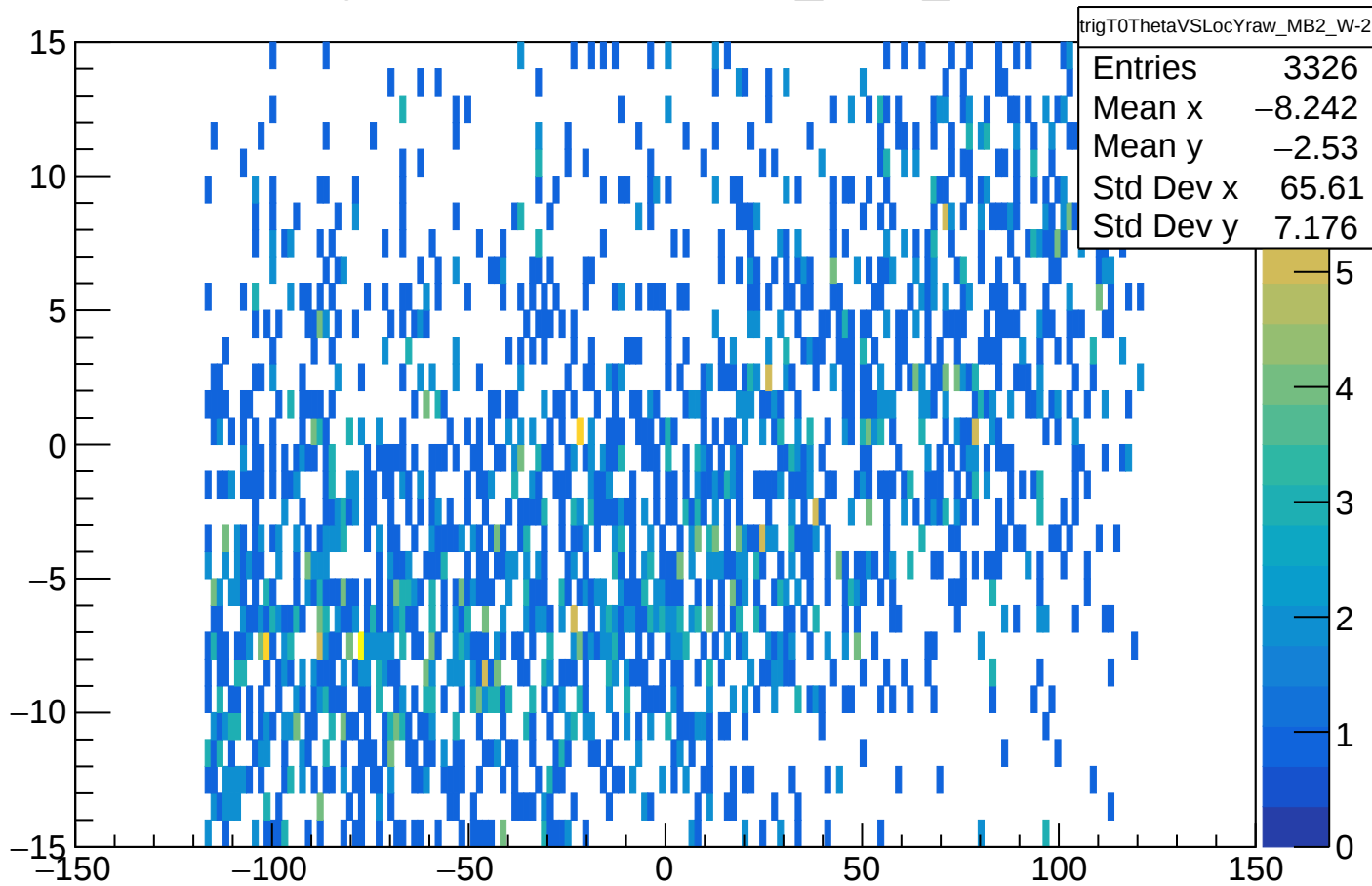
trigT0ThetaVSLocYraw_MB2_W-2
