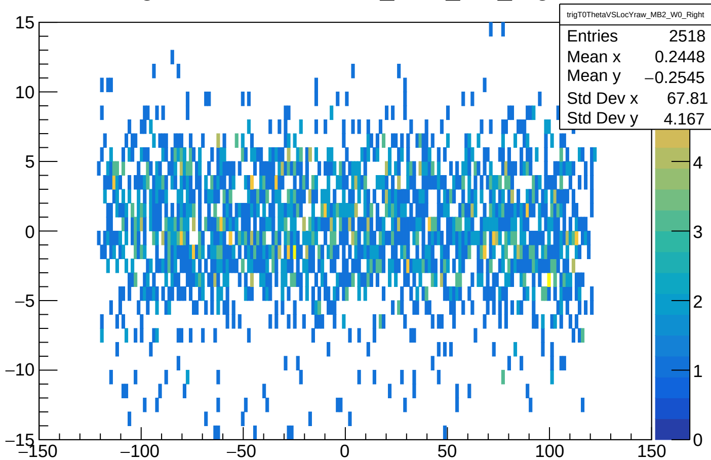
trigT0ThetaVSLocYraw_MB2_W0_Right
