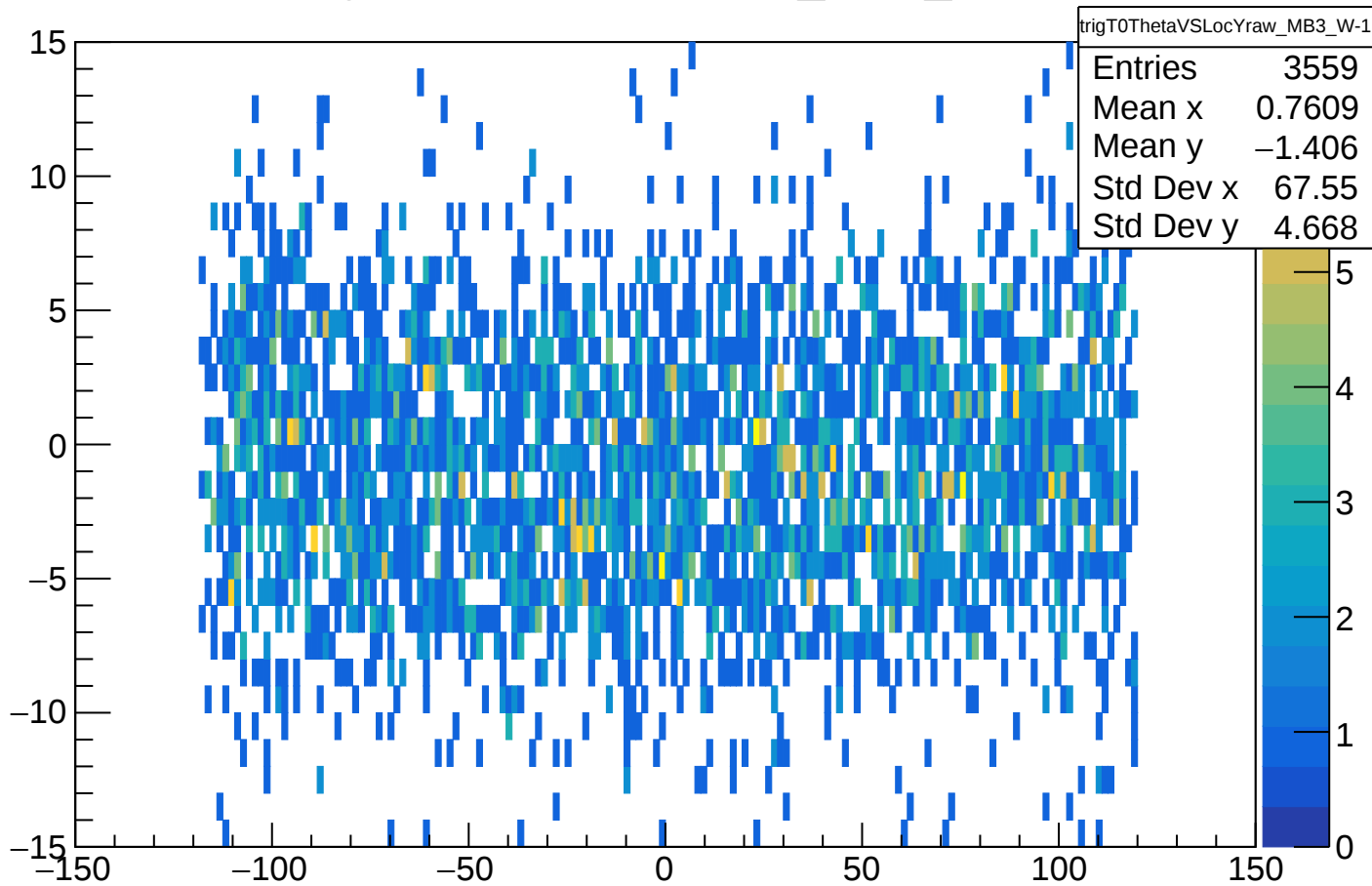
trigT0ThetaVSLocYraw_MB3_W-1
