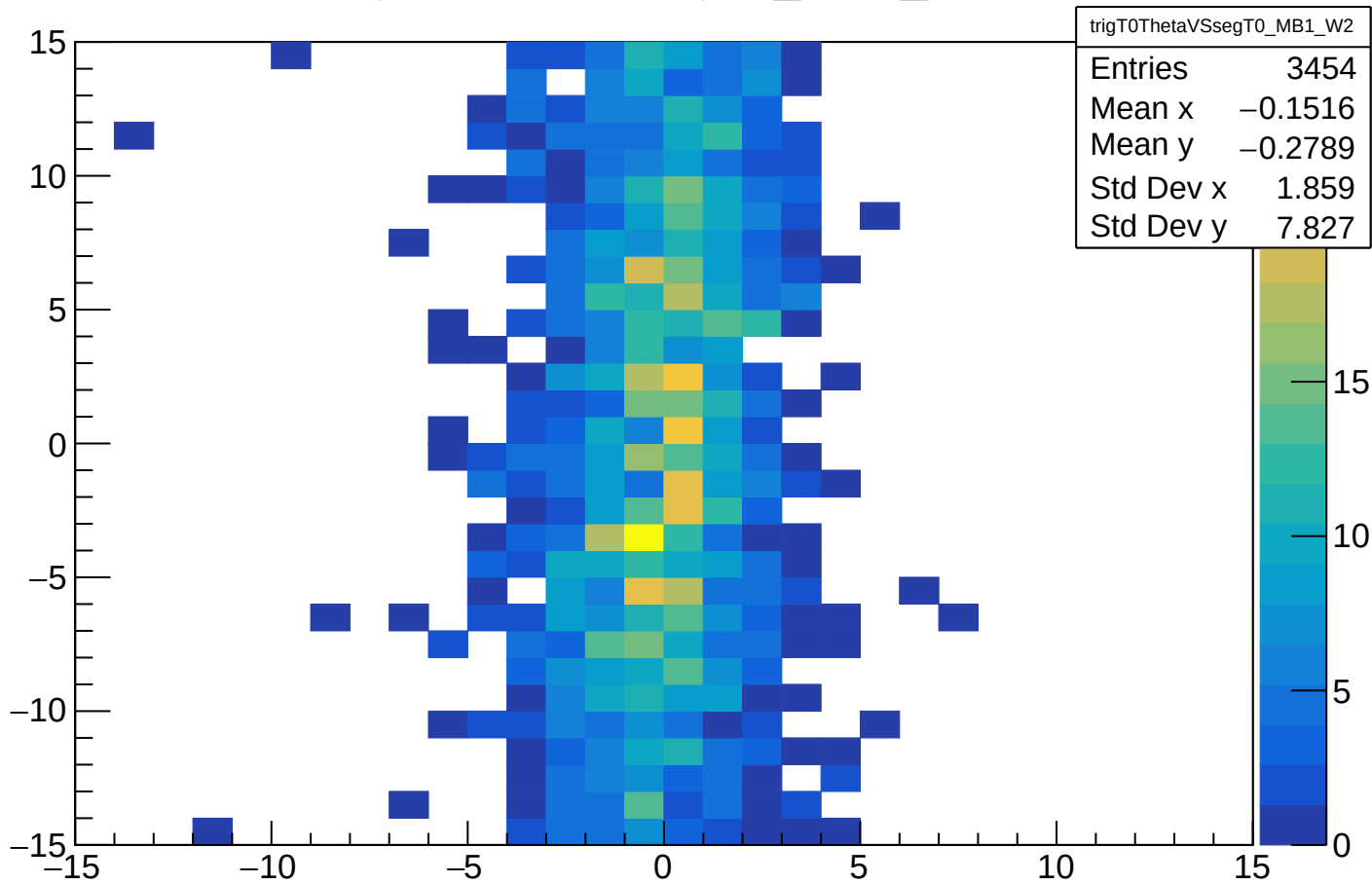
trigT0ThetaVSssegT0_MB1_W2
