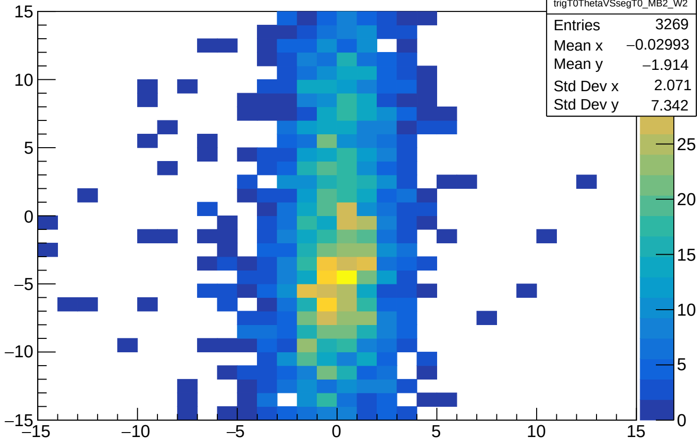
trigT0ThetaVSssegT0_MB2_W2
