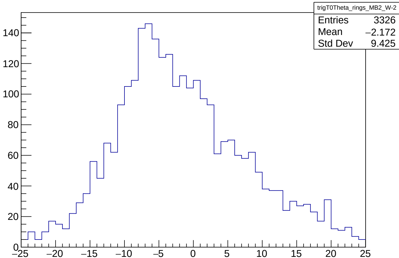
trigT0Theta_rings_MB2_W-2
