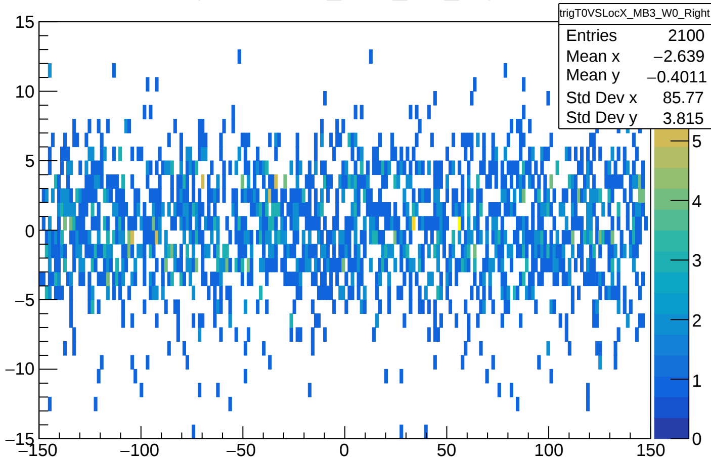
trigT0VSLocX_MB3_W0_Right
