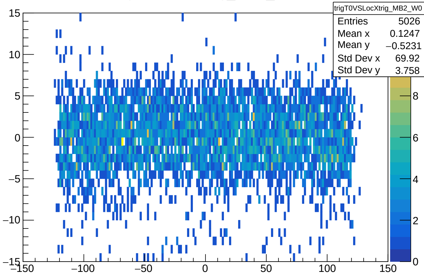
trigT0VSLocXtrig_MB2_W0
