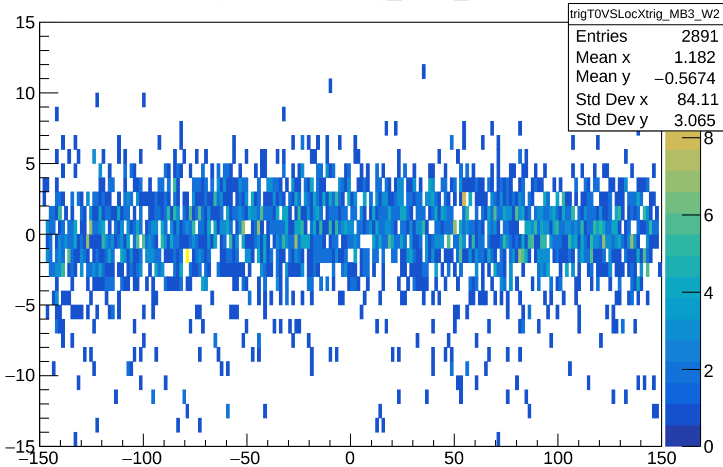
trigT0VSLocXtrig_MB3_W2
