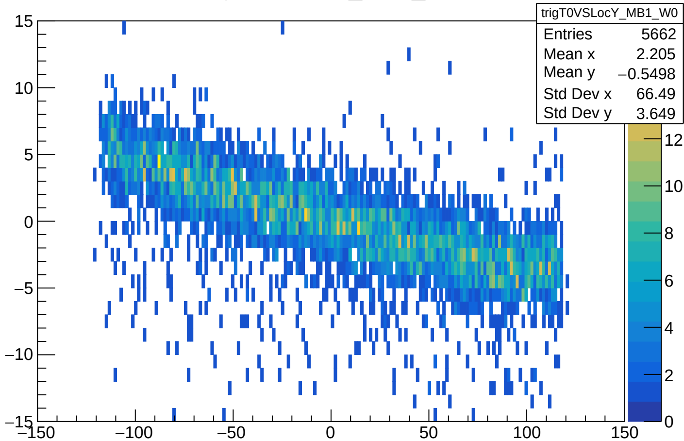
trigT0VSLocY_MB1_W0
