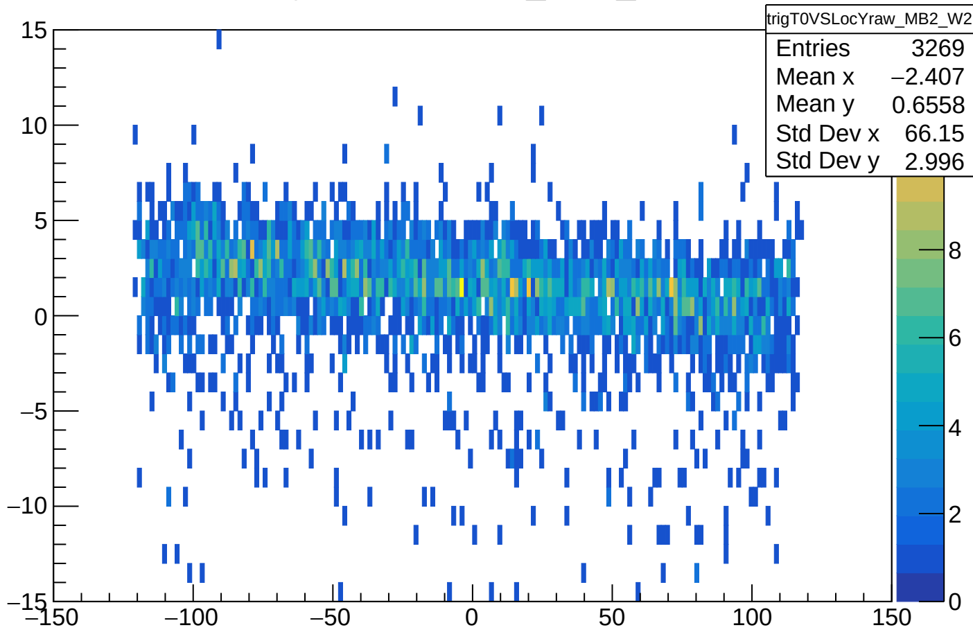
trigT0VSLocYraw_MB2_W2
