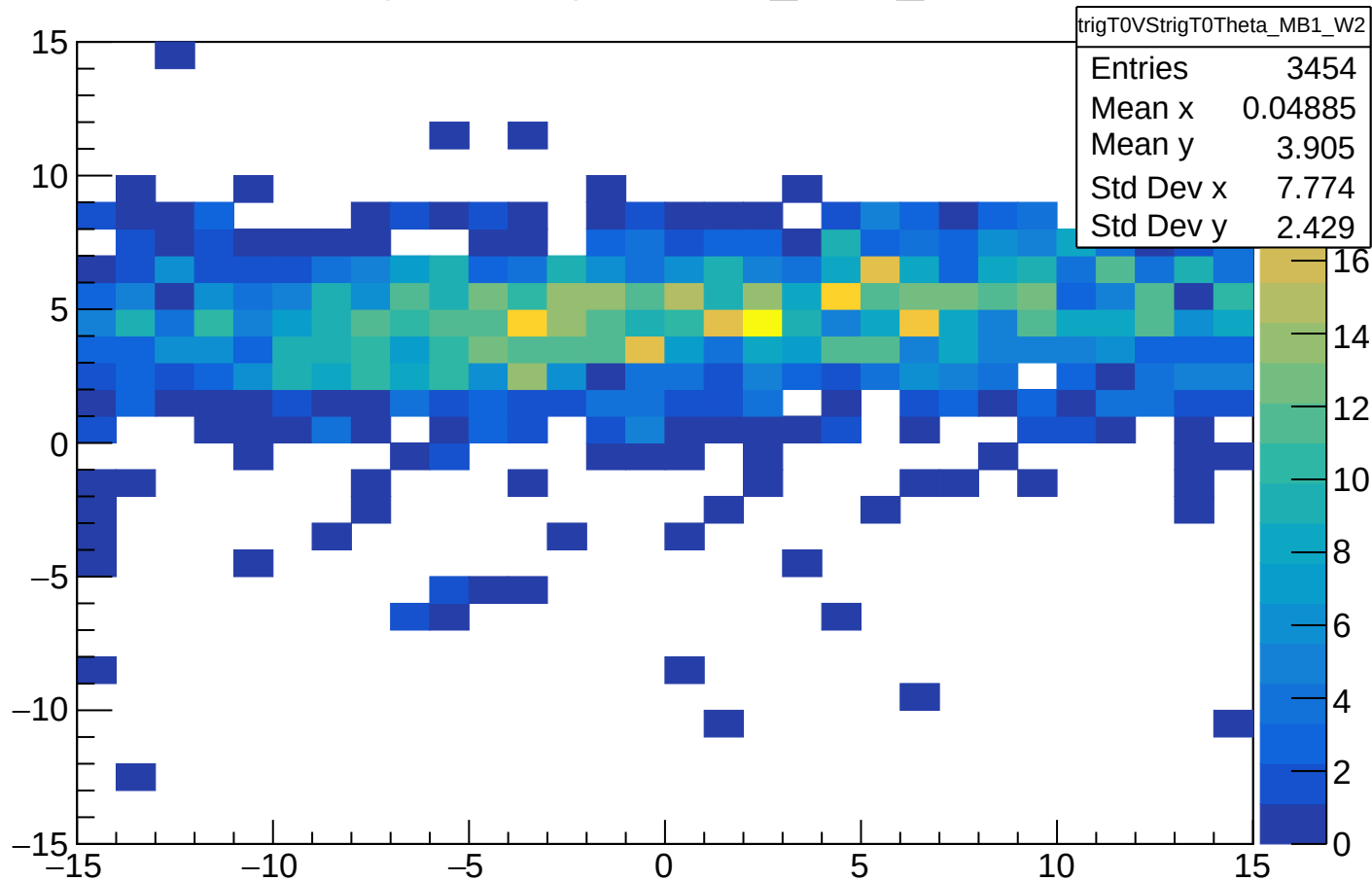
trigT0VStrigT0Theta_MB1_W2
