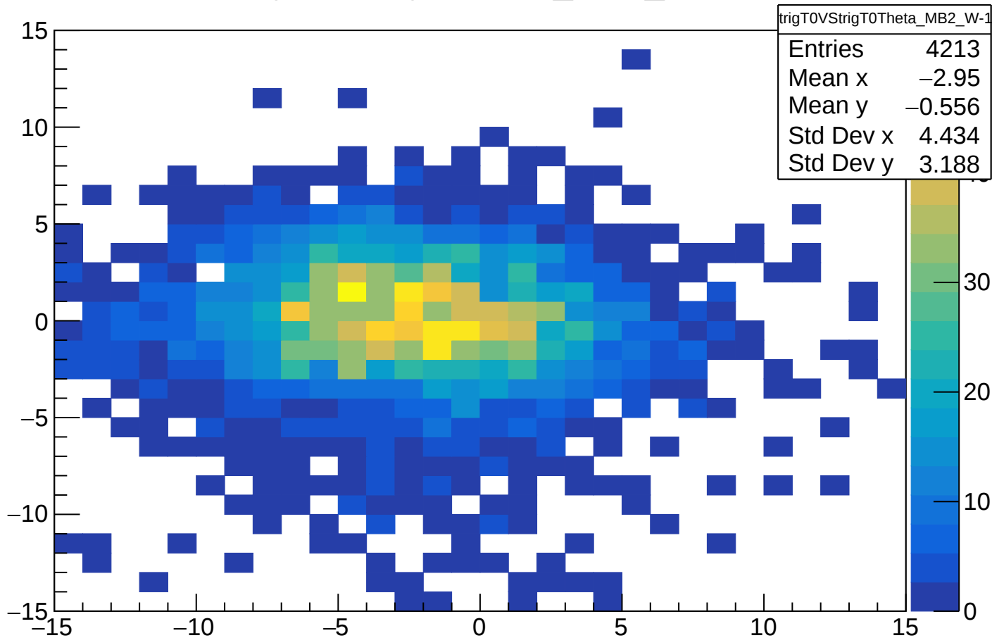
trigT0VStrigT0Theta_MB2_W-1
