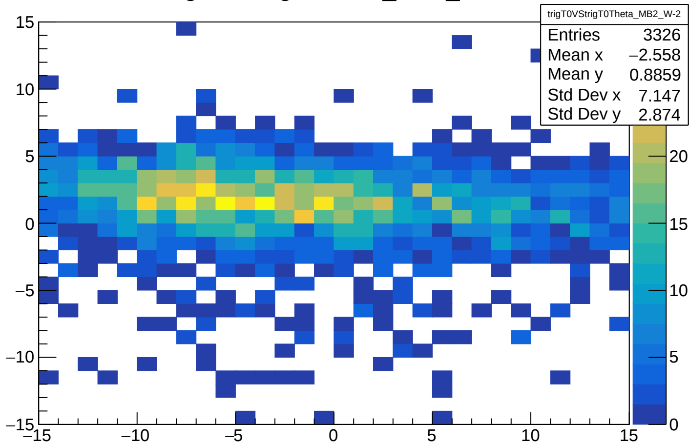
trigTOVStrigT0Theta_MB2_W-2
