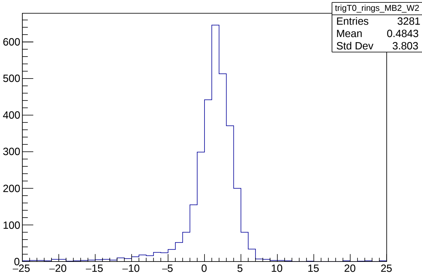
trigT0_rings_MB2_W2
