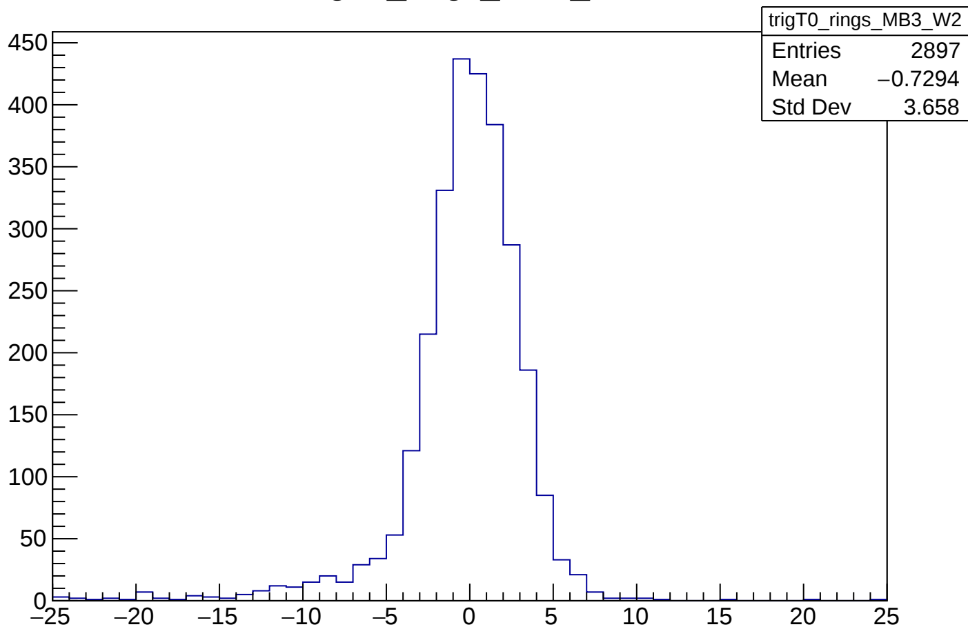
trigT0_rings_MB3_W2
