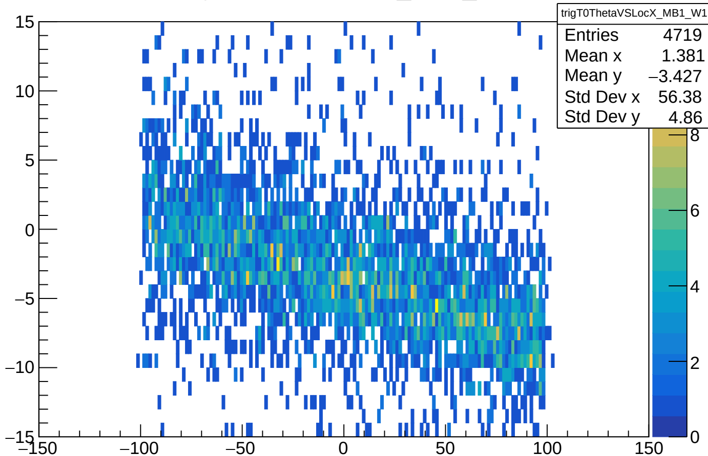
trigT0ThetaVSLocX_MB1_W1
