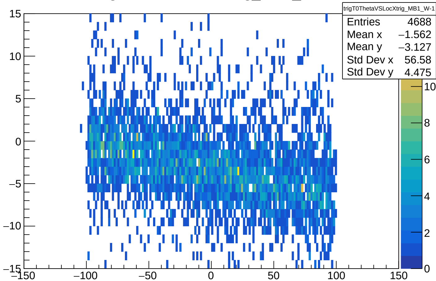
trigT0ThetaVSLocXtrig_MB1_W-1
