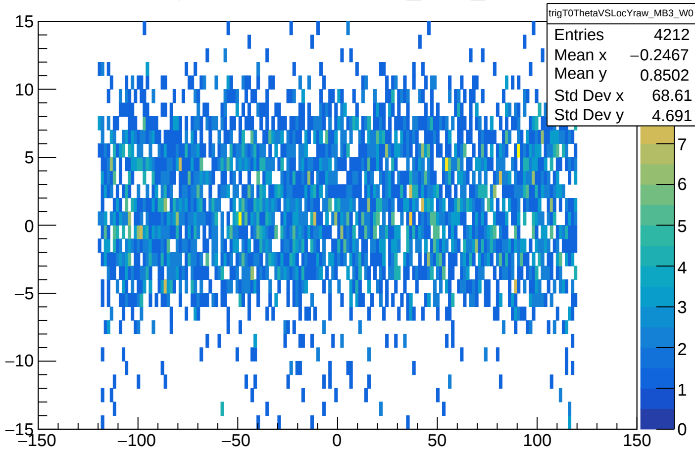
trigT0ThetaVSLocYraw_MB3_W0
