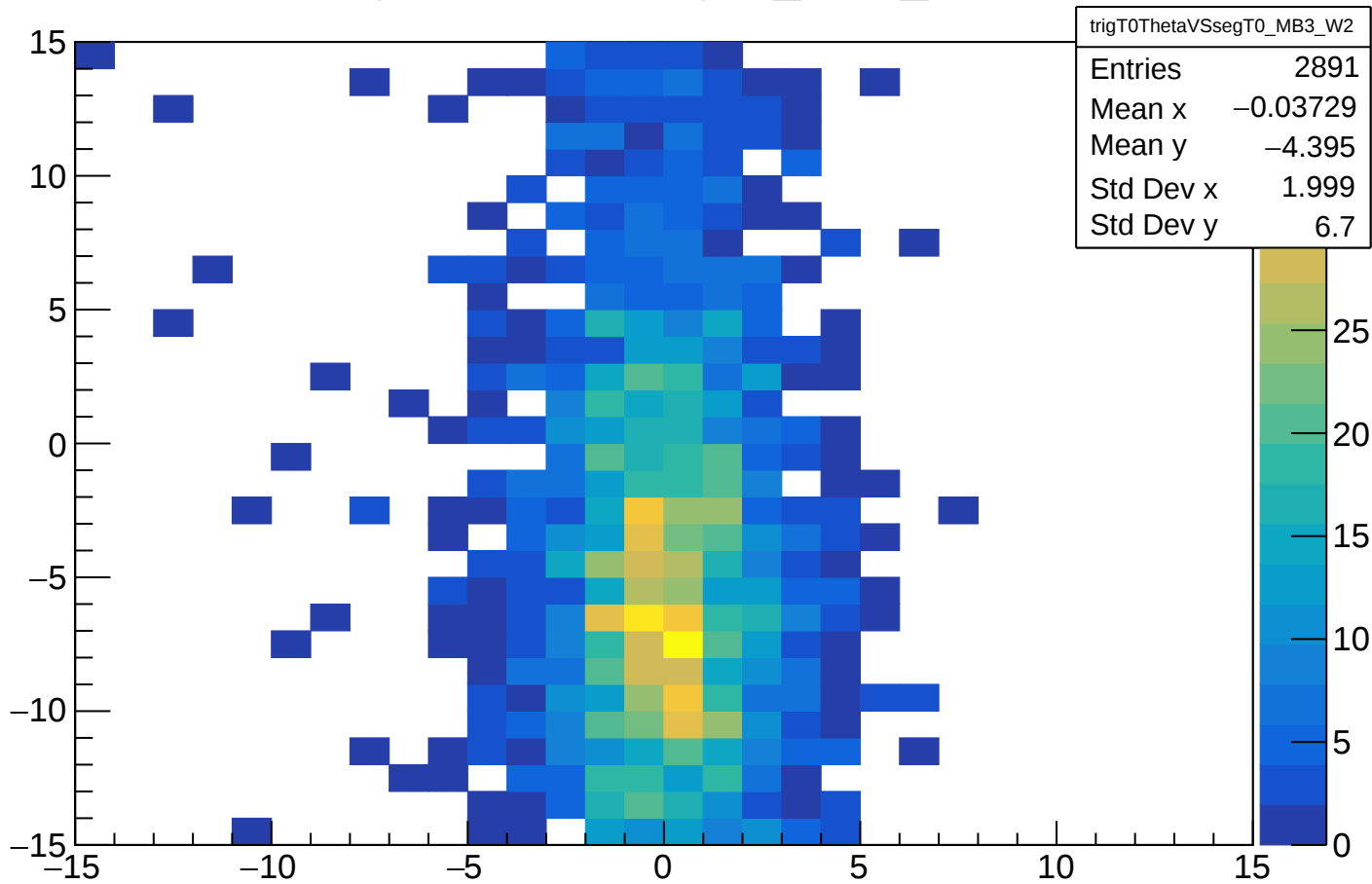
trigT0ThetaVSssegT0_MB3_W2
