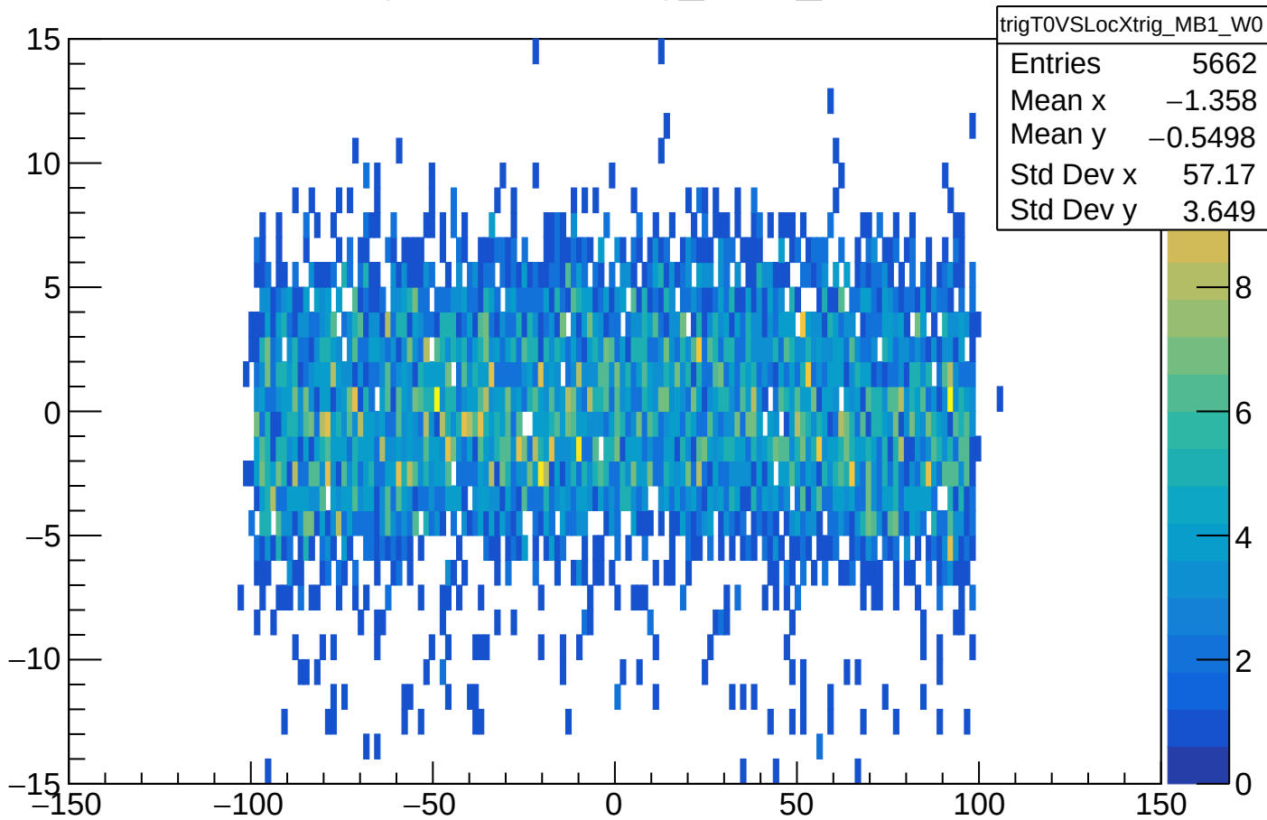
trigT0VSLocXtrig_MB1_W0
