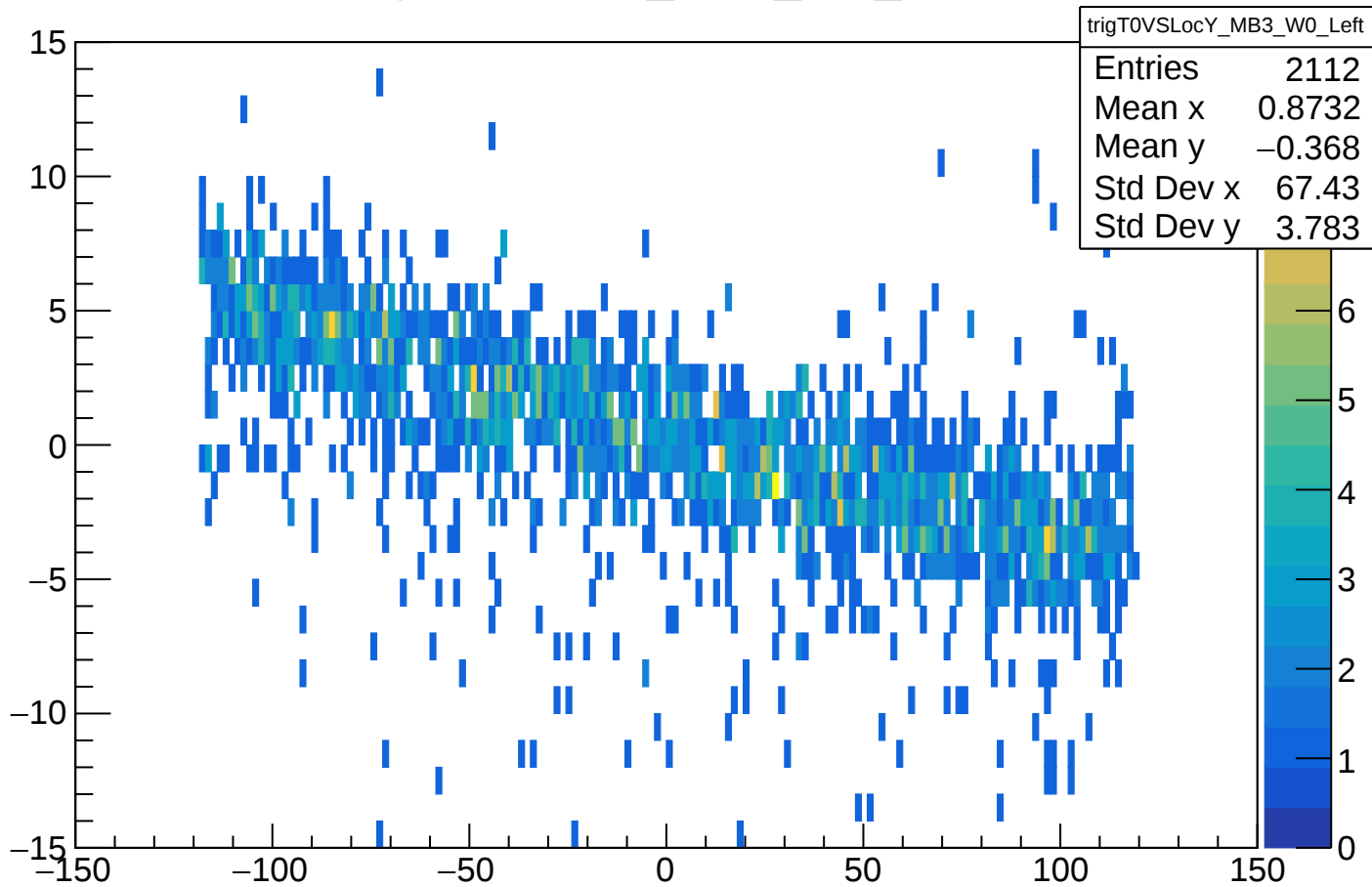
trigT0VSLocY_MB3_W0_Left
