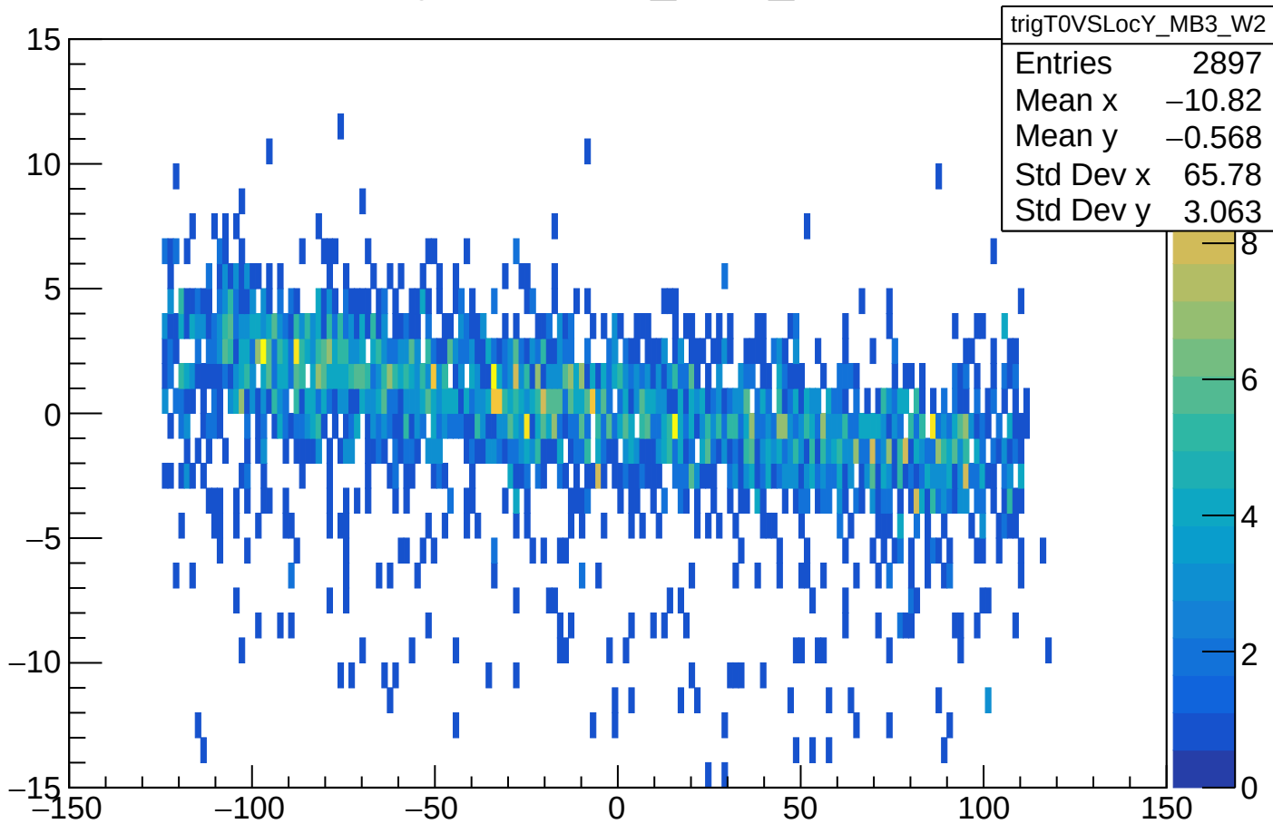
trigT0VSLocY_MB3_W2
