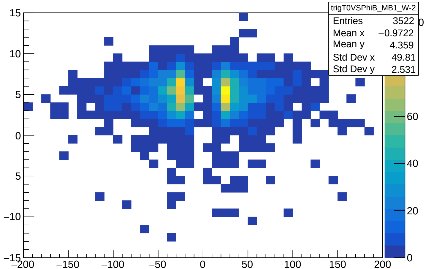
trigT0VSPhiB_MB1_W-2
