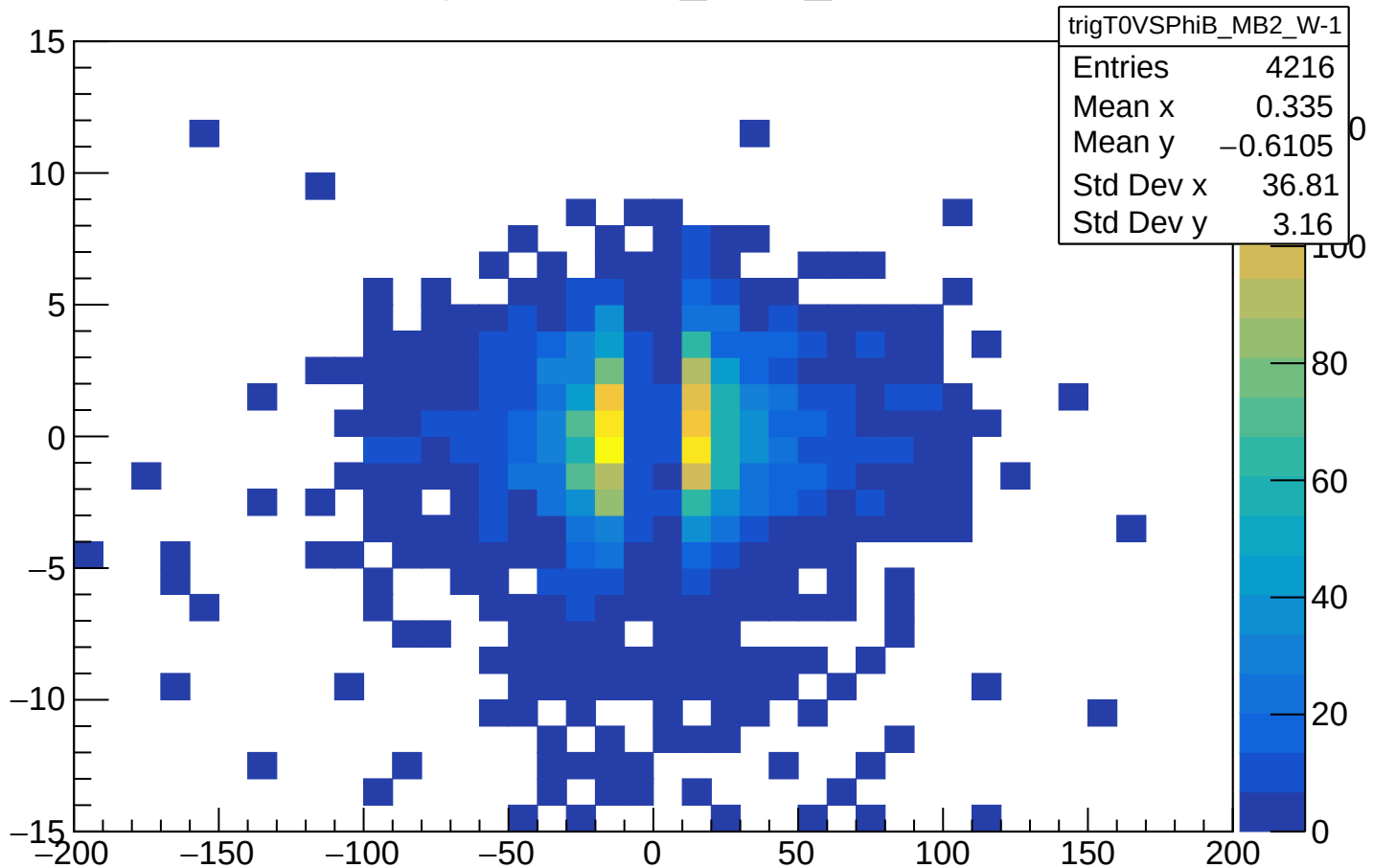
trigT0VSPhiB_MB2_W-1
