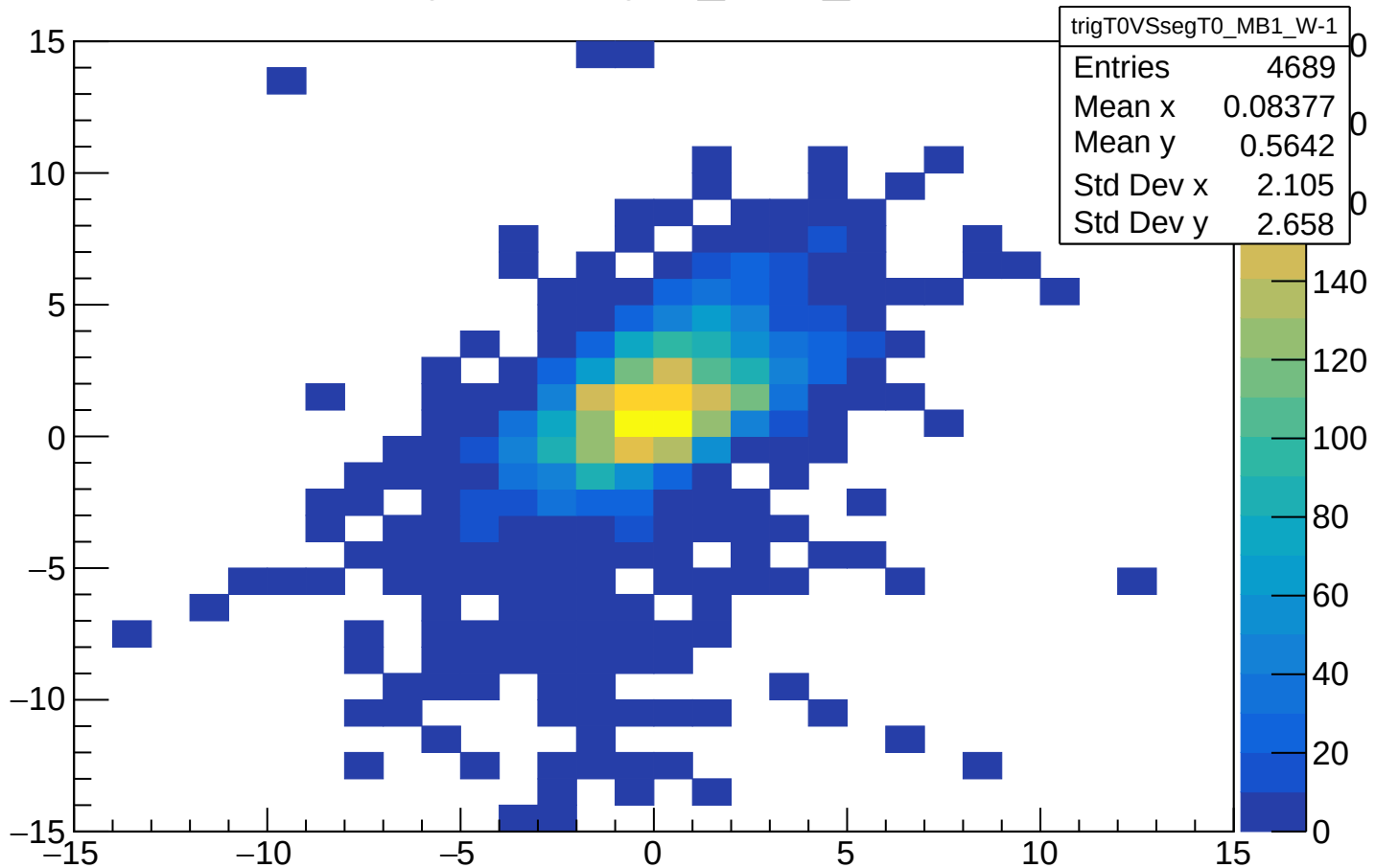
trigT0VSsegT0_MB1_W-1
