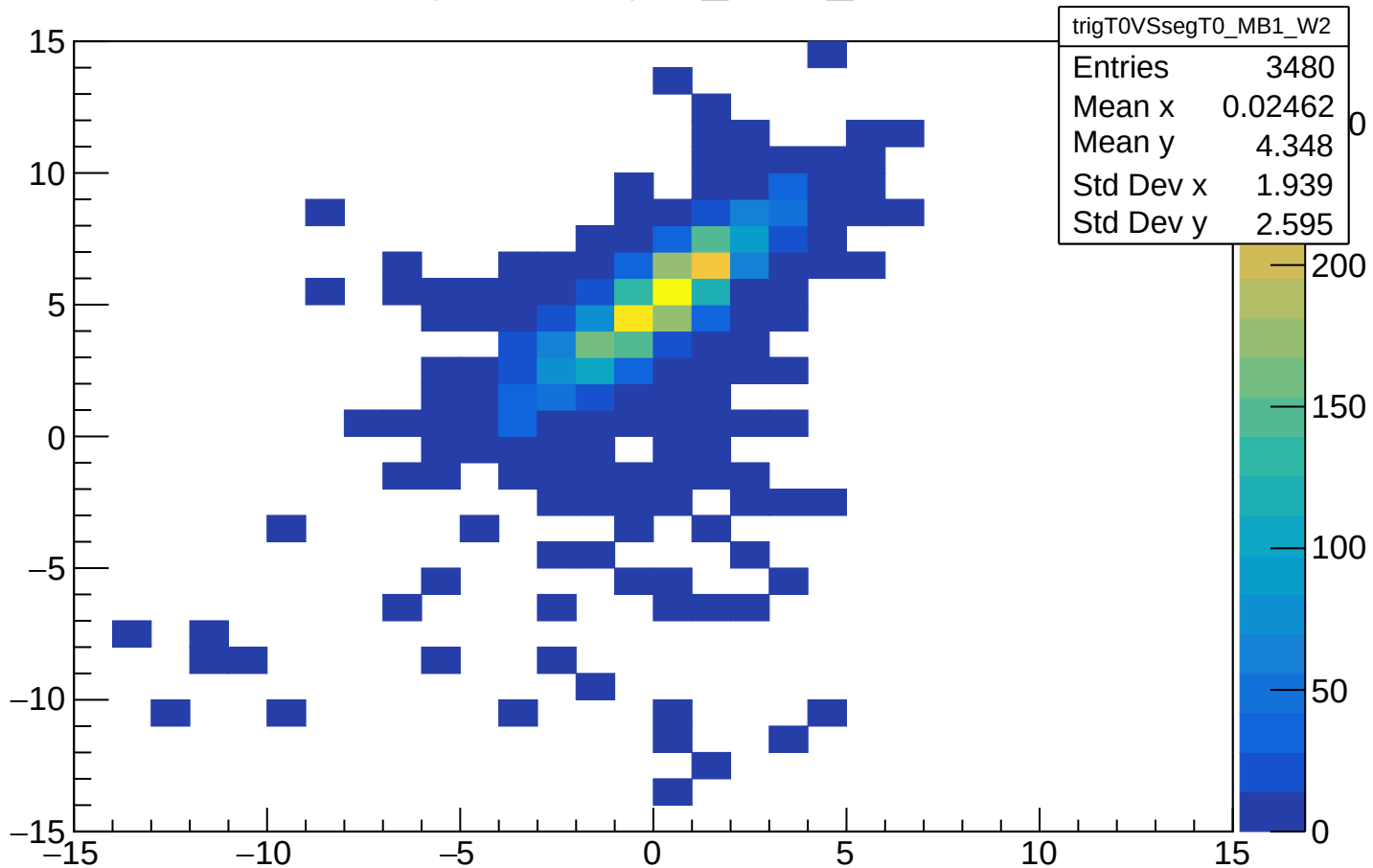
trigT0VSsegT0_MB1_W2
