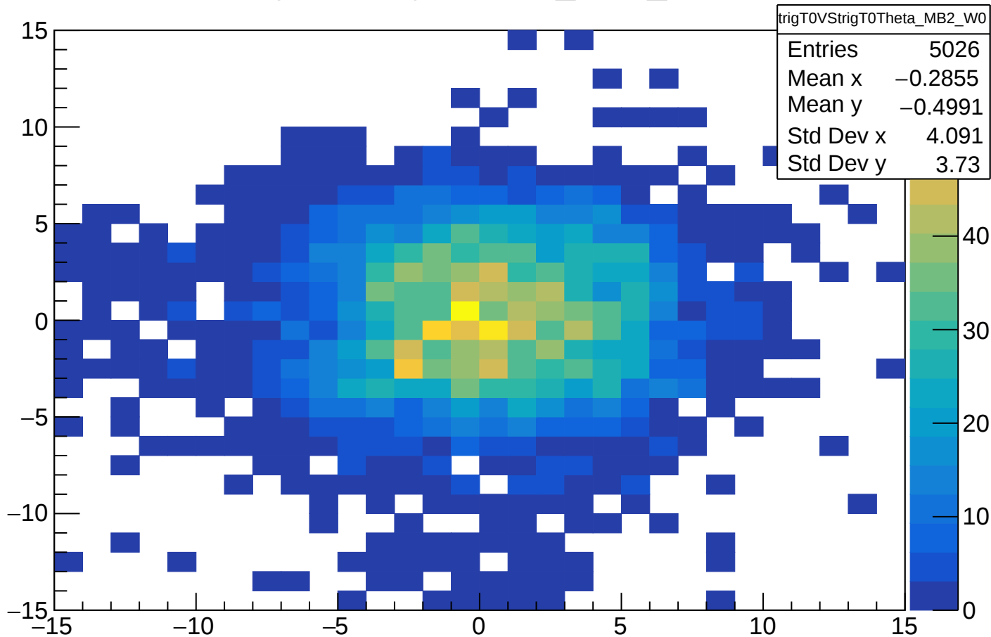
trigT0VStrigT0Theta_MB2_W0
