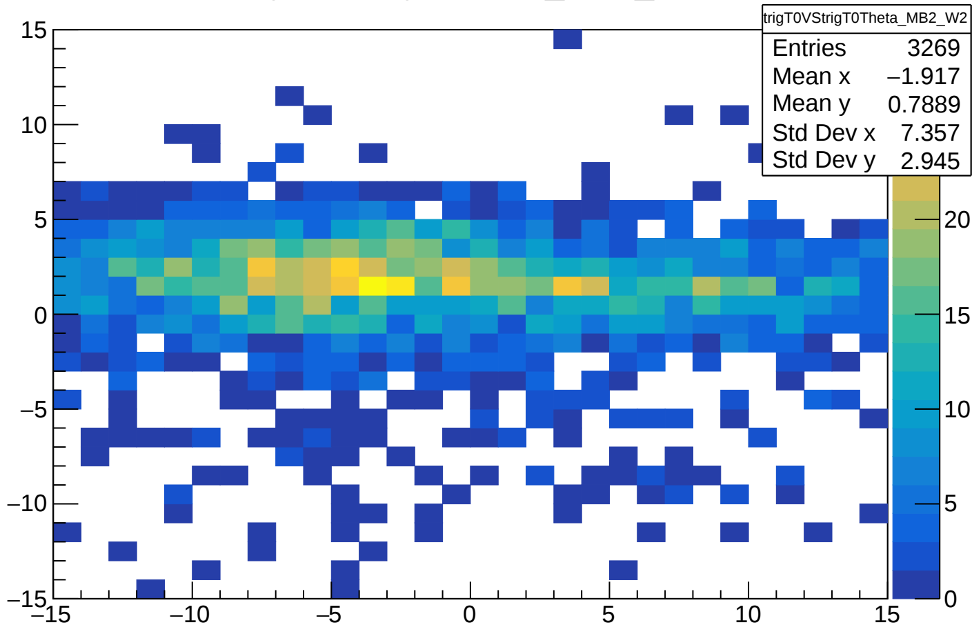
trigT0VStrigT0Theta_MB2_W2
